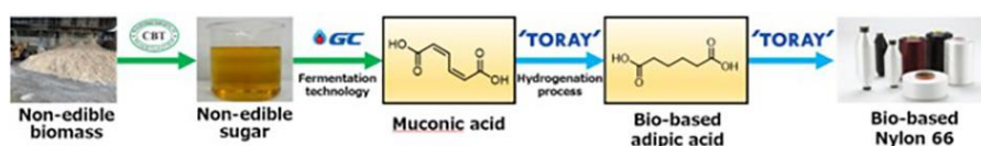
Fig 1. Procédé de fabrication du nylon 6,6 biosourcé
